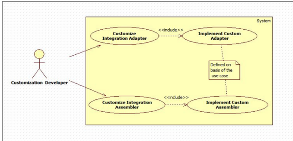
Figure 3–12 OCH Integration
